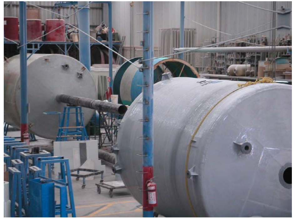
línea de ensamble y embobinado de cilindros
